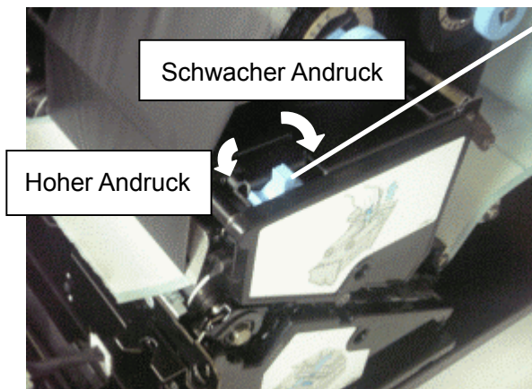
Kopfdruck Einstellhebel
